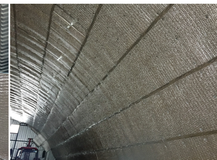
Монтаж отражательной теплоизоляции ПЕНОФОРМ® тип В толщиной 30 мм к внутренней поверхности бескаркасного ангара
