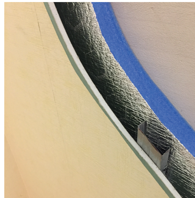
Внутреннее утепление ограждающей конструкции системы с замкнутым воздушным зазором и отражательной массивной теплоизоляцией из вспененного полиэтилена ПЕНОФОРМ®.
